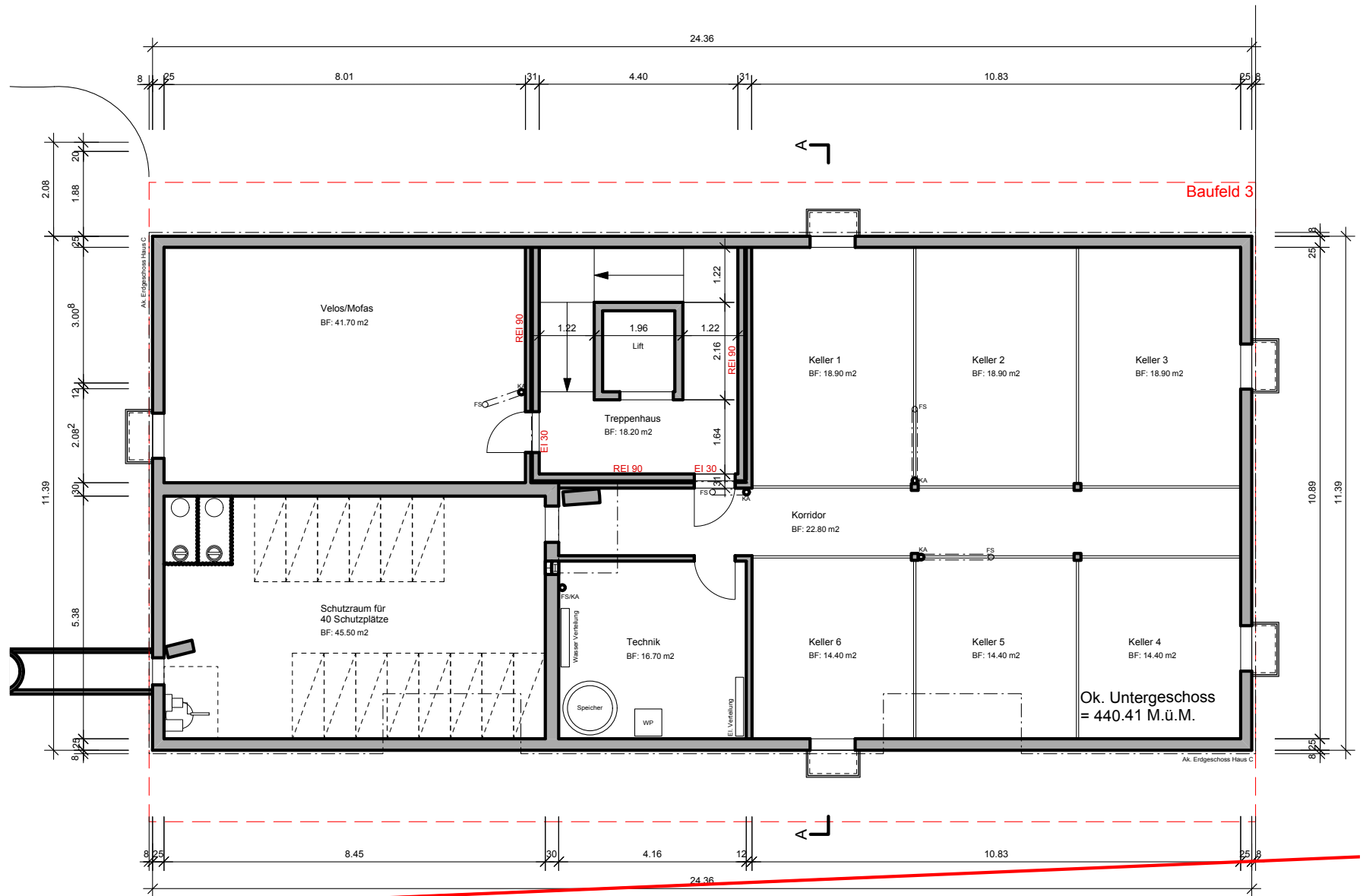
Grundriss Untergeschoss
